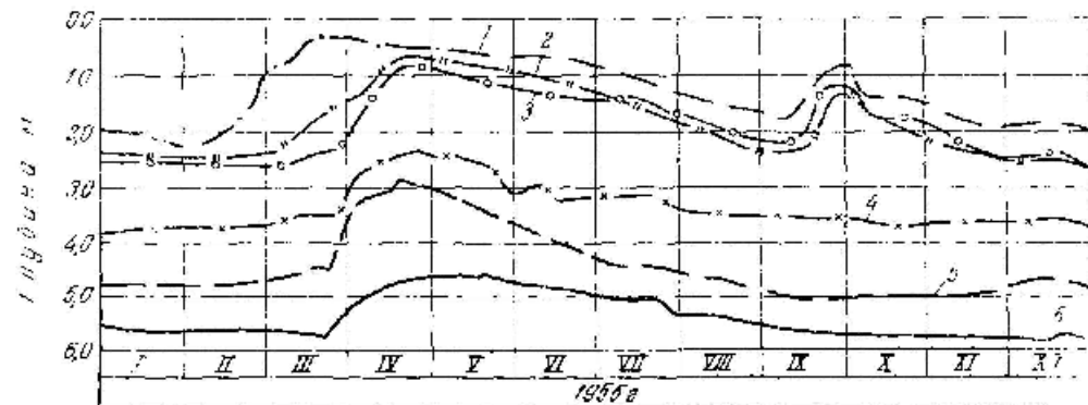
Рис. 54. График колебания уровня подземных вод Куинского гранитного массива скважины: 1—23; 2—14; 3—19; 4—39; 5—18; 6—22
