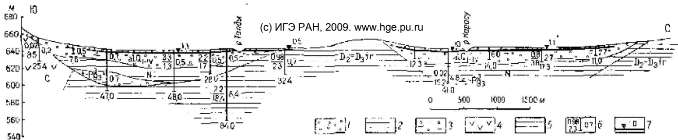
Рис. 37. Гидрогеологический разрез низовья долины р. Талды (составила Л. А. Рыбалтовская)
