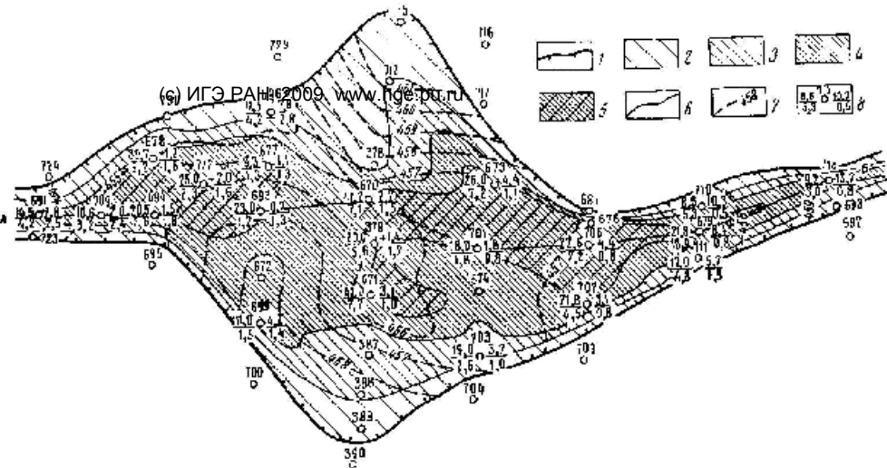
Рис. 29 Гидрогеологическая карта водоносного горизонта верхнеолигоценных отложений Молодцовского участка долины р. Нуры (составила Э. Д. Кузьмина по материалам П. И. Савчука, Ж. Букетова)
