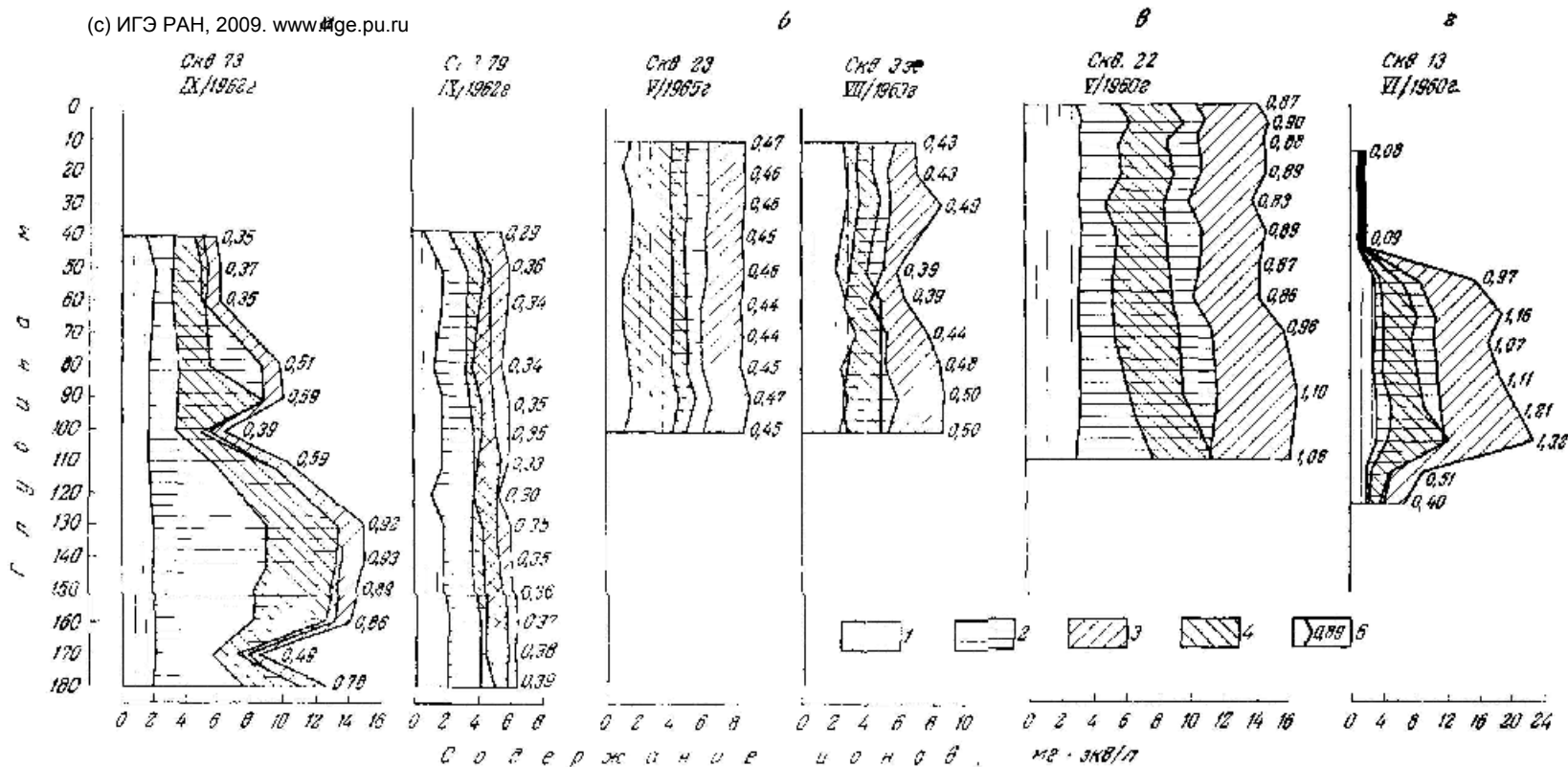
Рис. 24. Графики вертикальной гидрохимической зональности подземных вод карбонатных фаменских и турнезских отложений: а - Уртакашлыкская синклиналь, б - Эскуленская антиклиналь, в - Жанаевская антиклиналь, г - Айдооская антиклиналь, содержание ионов (мг·л/л): 1 - \text{CO}_3^{2-} , 2 - \text{SO}_4^{2-} , 3 - \text{Cl}^- , 4 - \text{Mg}^{2+} , 5 - \text{Ca}^{2+} . Содержание \text{Ca}^{2+} отбрасывается от нуля. График б - минерализация воды (г/л).
