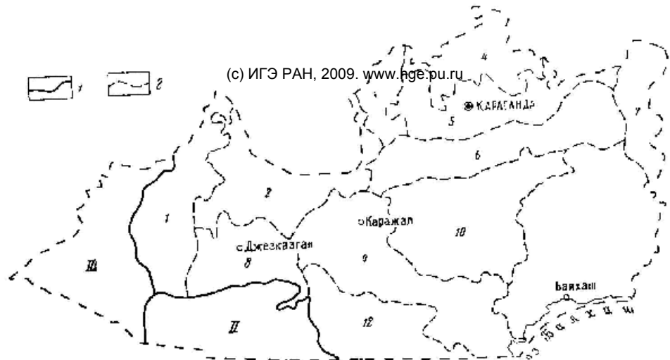
Рис. 19. Схема гидрогеологического районирования Карагандинской области
