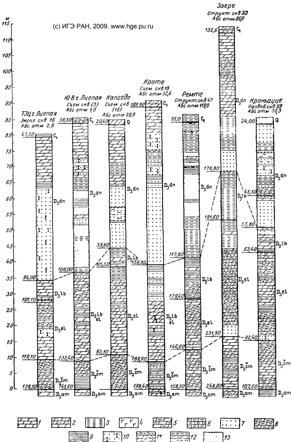
Рис. 7. Разрезы фамениского яруса.
