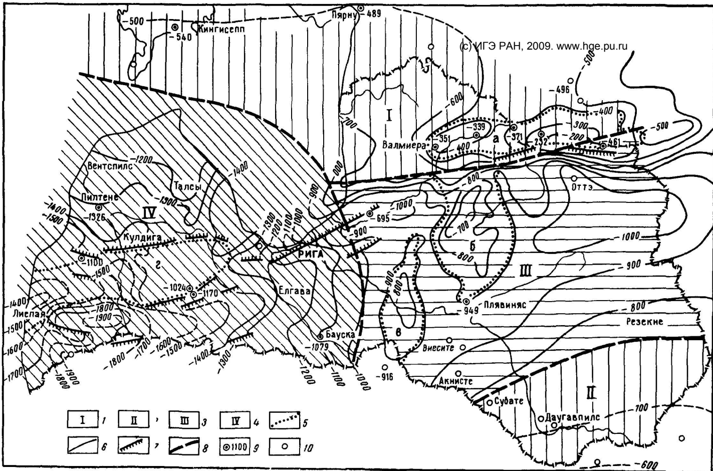
Рис 6 Тектоническая схема Латвийской ССР
