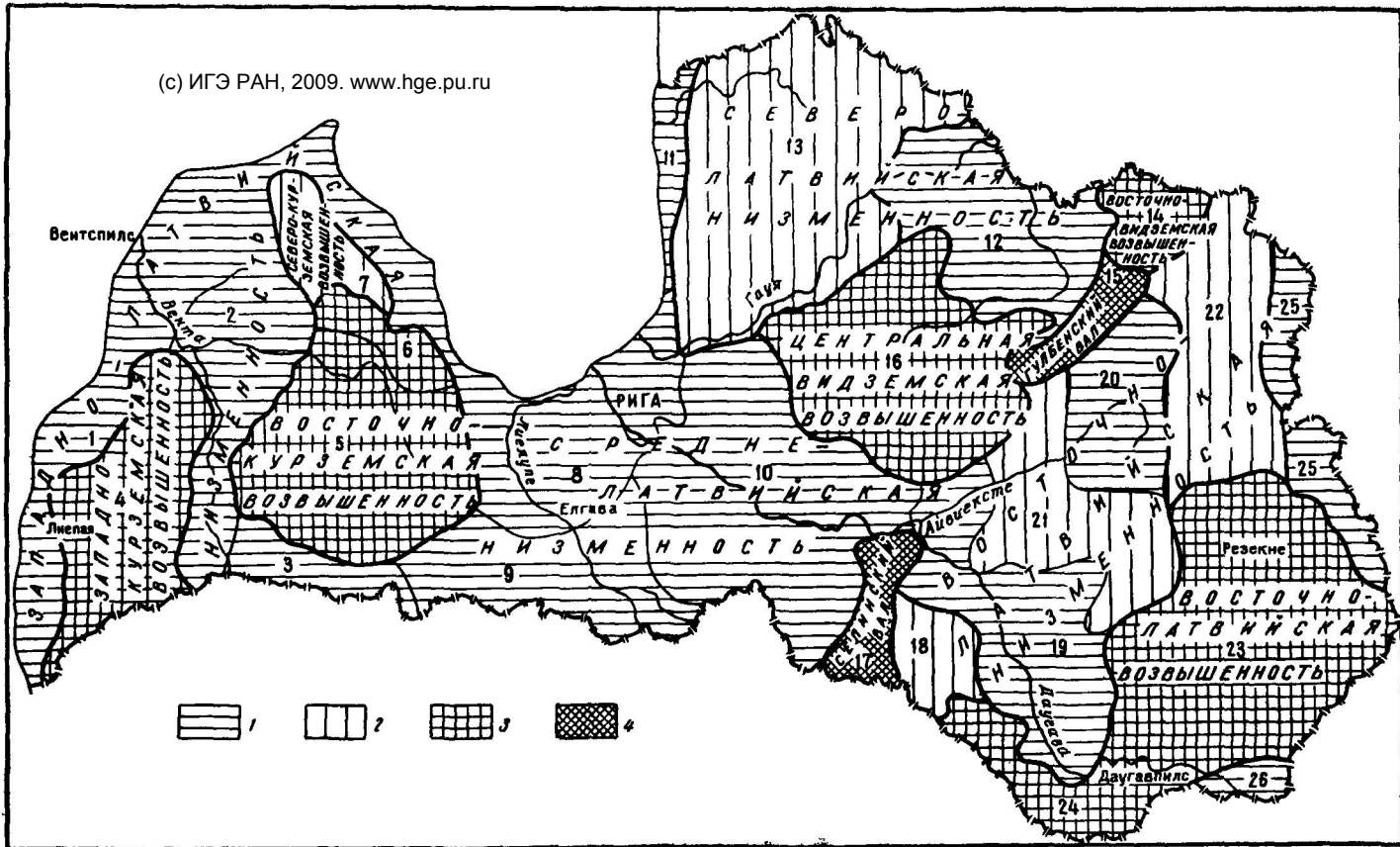
Рис. 4. Схематическая карта геоморфологического районирования Латвийской ССР (по А И Яунпутниньшу, 1961). 1 — низменности, 2 — поднятия, 3 — возвышенности, 4 — валообразные возвышенности (валы)
