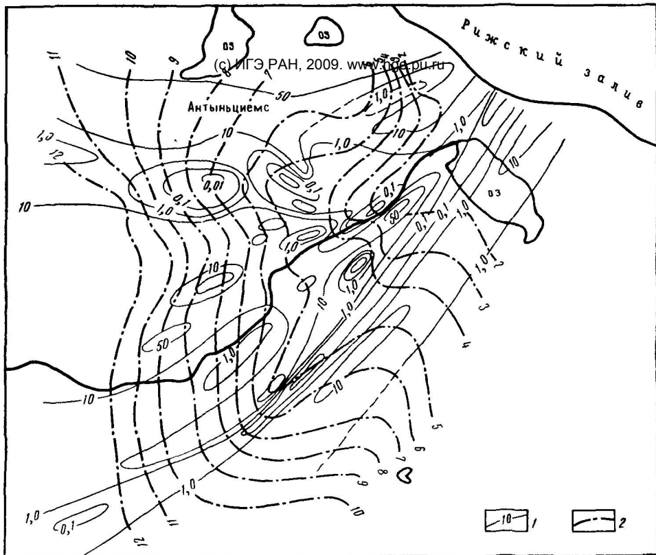
Рис. 30 Схема гидроизопез и содержания сульфатредуцирующих бактерий в водах верхней части саргаевского водоносного горизонта района Кемерово
