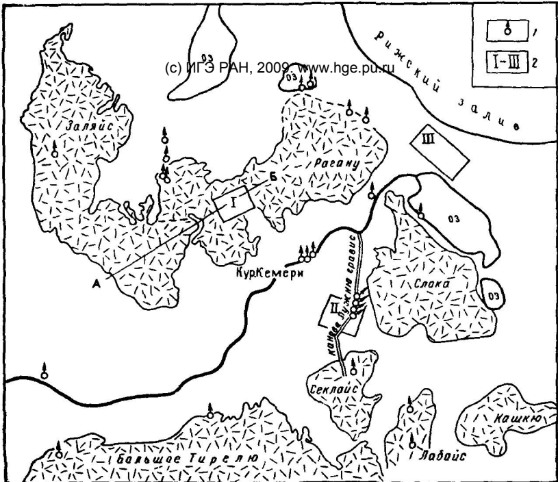
Рис. 27. Схема гидрографической сети в районе Кемерови 1 — источники; 2 — участки с повышенным содержанием H 2 S
