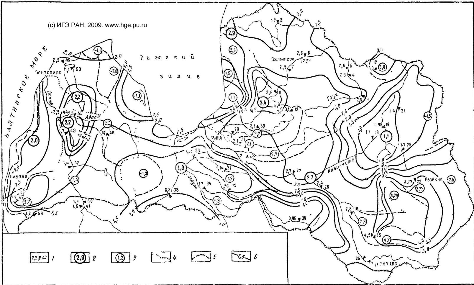
Рис 22 Схематическая карта изолиний модулей подземного стока — разгрузки в реки и в море зоны интенсивного водообмена 1 — створ замеров расхода реки, справа — его номер, слева — значение модуля подземного стока в реку в л/сек с 1 км 2 , 2 — центр тяжести и модуль подземного стока для бассейна основной реки, 3 — центр тяжести и модуль подземного стока для речного бассейна второго порядка, 4 — граница бассейна основной реки, 5 — граница бассейна притока или характерного участка стока, 6 — изолиния модуля стока
