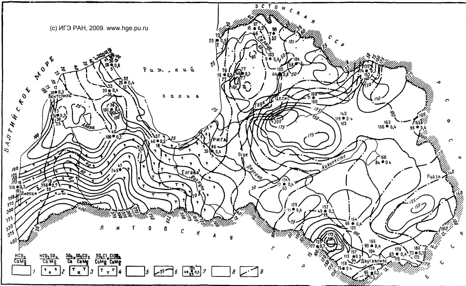
Рис 14 Схематическая карта глубин залегания кровли, гидроизопьез и химического состава швентойско тартуского водоносного комплекса 1 — гидрокарбонатно кальциево магниевые воды с минерализацией до 0,5 г/л, 2 — гидрокарбонатно сульфатно кальциево магниевые воды с минерализацией 0,5—1 г/л, 3 — сульфатно гидрокарбонатно кальциево магниевые воды с минерализацией до 3 г/л, 4 — сульфатно хлоридно кальциево магниевые воды с минерализацией 1—3,0 г/л, 5 — участки с невыявленным химическим составом 6 — изолинии глубин залегания кровли от поверхности земли, проведенные через 25 м 7 — скважина цифра сверху — номер по каталогу, слева — глубина залегания кровли от поверхности земли в м справа — величина минерализации в г/л внизу — пьезометрический уровень в абс отн в м, 8 — контур распространения вод с различной минерализацией 9 — гидроизопьезы, проведенные через 20 м Величина минерализации показана для верхней части комплекса
