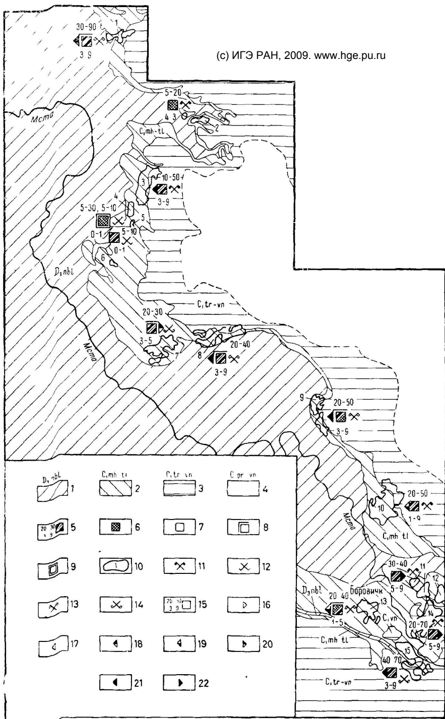
Рис. 31. Гидрогеологическая карта-схема месторождения огнеупорных глин Боровичско-Любытинского горнопромышленного района (по материалам И. В. Котлуковой, 1963 г., Е. Д. Остромейки и др., дополнено И. А. Алексеевой, 1963 г)
