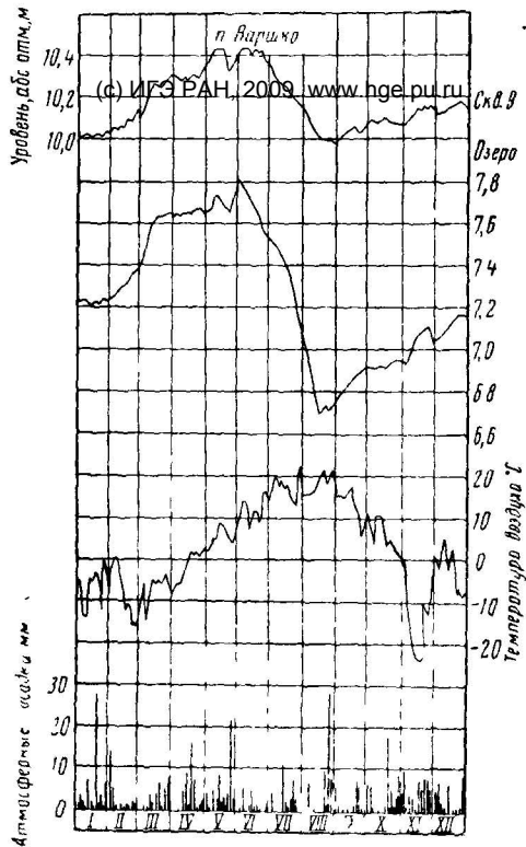
Рис 19 Типовые графики естественного режима уровня подземных вод нижнекембрийских отложений (составила П. М. Гасс, 1964 г по данным Северо-Западной гидрогеологической станции)
