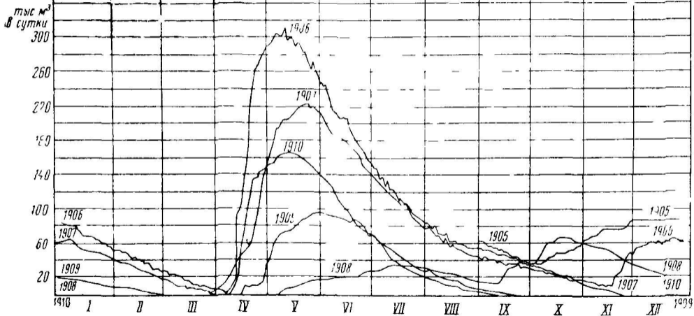
Рис 18 График колебания расхода карстовых источников в верховьях р Пудости за 1905–1910 гг. (по данным Н. Ф. Погребова, 1913 г.)
