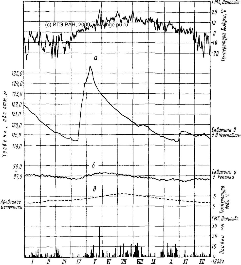
Рис 17. Графики колебания уровня и температуры воды ордовикского водоносного комплекса в зависимости от гидрометеорологических условий (по данным Северо-Западной гидрогеологической станции, 1958 г.)
