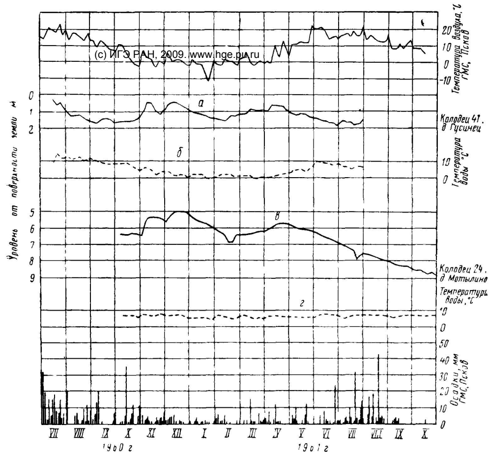
Рис 16 График колебания уровня и температуры подземных вод четвертичных и верхнедевонских отложений в зависимости от гидрометеорологических условий, по данным И. М. Вербовой (А. И. Шмаенок и др., 1963 г.)
