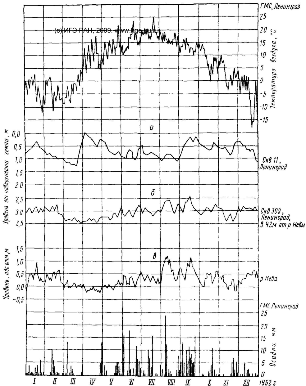
Рис 15. Графики колебания уровня подземных вод четвертичных отложений в зависимости от гидрометеорологических условий и уровня р Невы (по данным Северо-Западной гидрогеологической станции, 1962 г)
