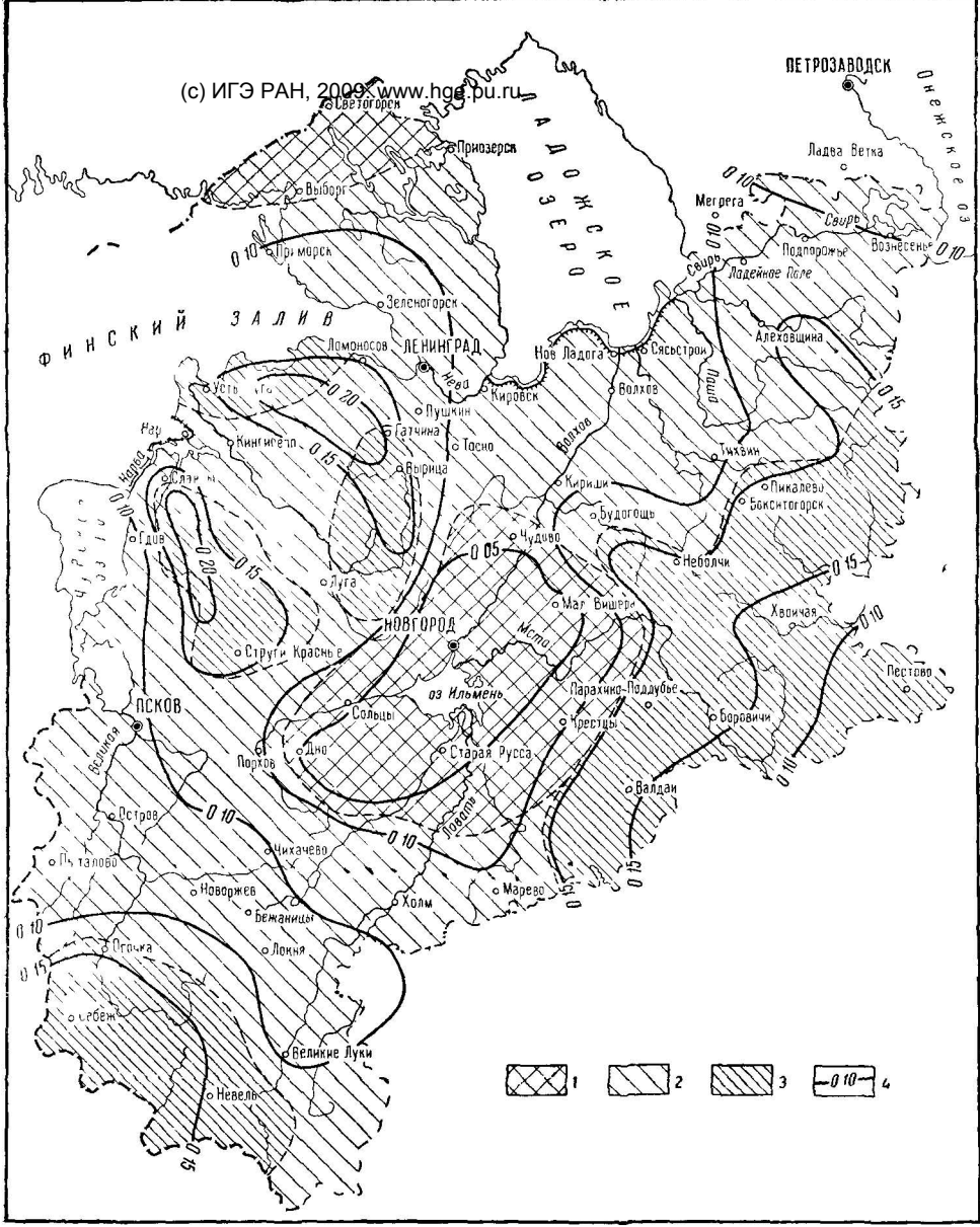
Рис. 13. Карта-схема коэффициентов подземного стока в реки (в долях единицы), величин подземного стока (в процентах от общего речного стока) по материалам карты подземного стока в Европейской части СССР, 1963 г) 1 — подземный сток составляет 10—20% от общего речного стока; 2 — 20—30%; 3 — 30—40%; 4 — изолинии коэффициента подземного стока в долях единицы
