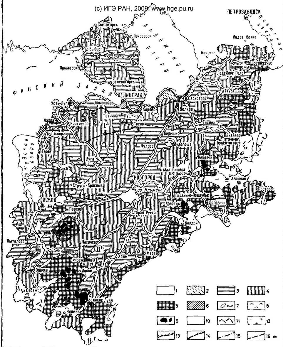
Рис. 6. Схематическая геоморфологическая карта (составил Д. Б. Малаховский, 1964 г.)
