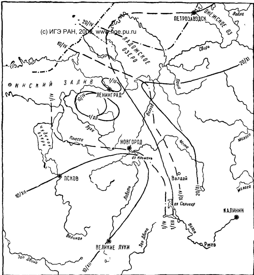
Рис. 4. Карта-схема изолиний средних многолетних дат начала и конца устойчивого снежного покрова (составила Е. В. Матлова)
