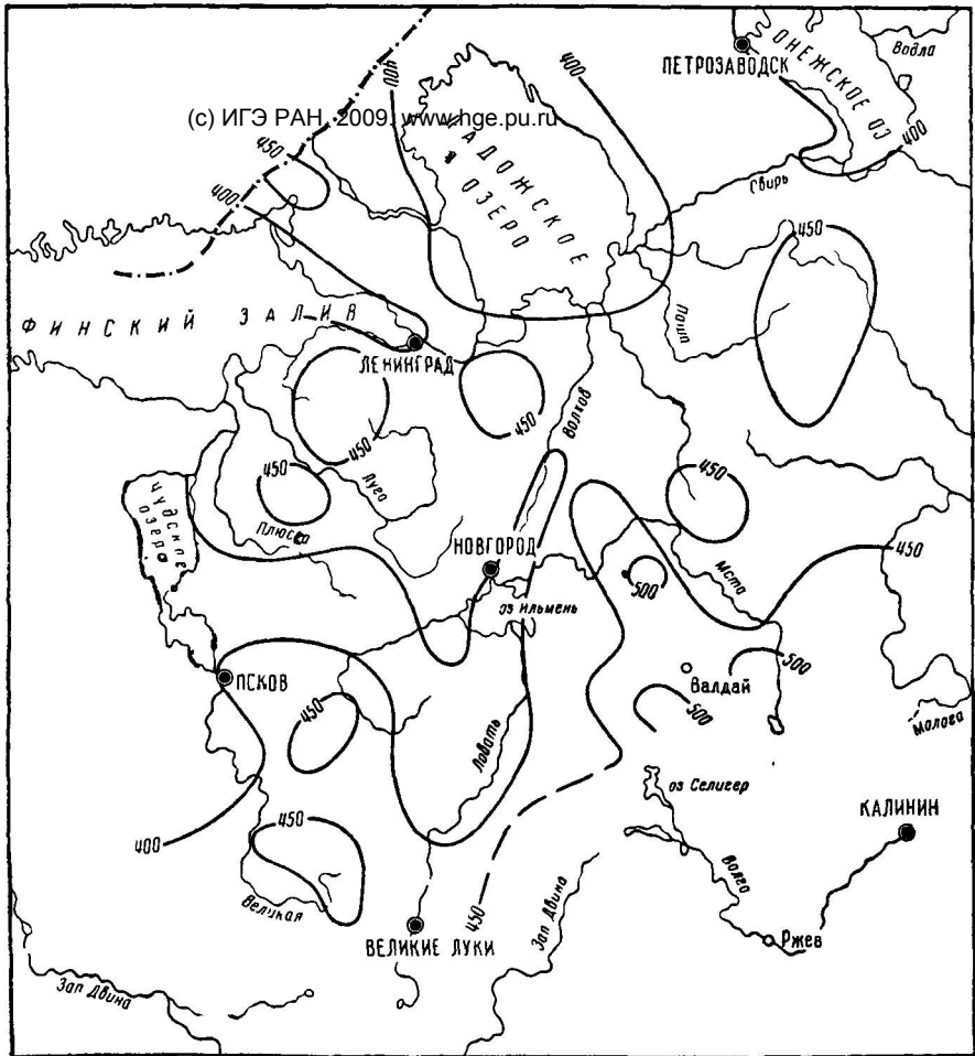
Рис. 3. Карта-схема изолиний средней многолетней суммы осадков за теплый период (апрель — октябрь) (составила Е. В. Матлова)
