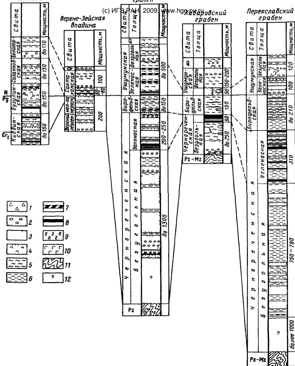
Рис. 8. Схема сопоставления опорных разрезов палеогеновых и неогеновых отложений Средне-Амурской, Амуру-Зейской и Верхне-Зейской впадин, по В. Г. Варнавскому
