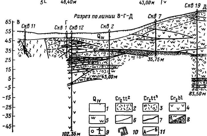
Рис 42 Геологическая карта и разрезы участка выхода Анненских термальных источников (четвертичный покров снят) Составили В В Кулаков и Н Н Егоров
