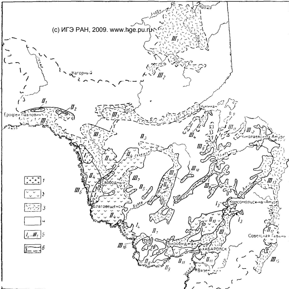
Рис. 37. Схематическая карта модулей эксплуатационных ресурсов подземных вод Хабаровского края и Амурской области. Составил И. Б. Райхлин
