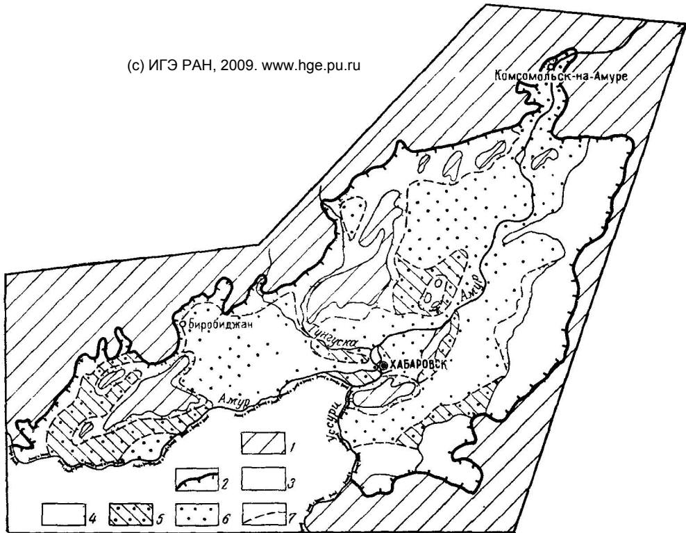
Рис. 30. Схема распространения железистых подземных вод в пределах Средне-Амурского артезианского бассейна
