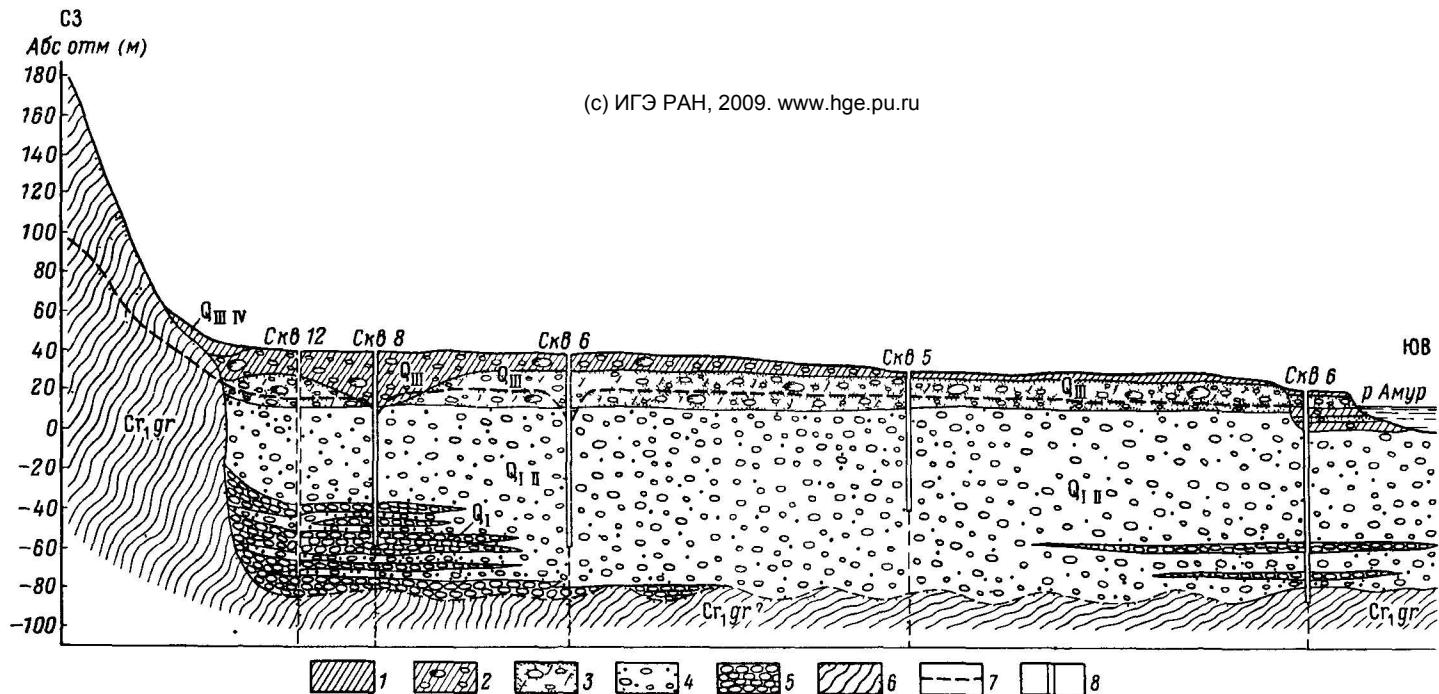
Рис. 25 Гидрогеологический разрез района г Комсомольска-на-Амуре (Хунгаринский бассейн второго порядка)
