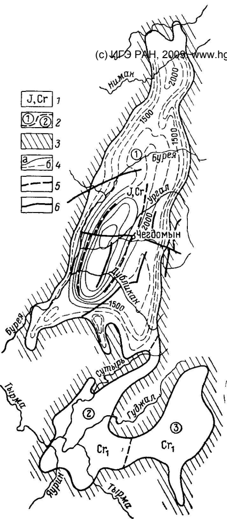
Рис. 21. Схема гидрогеологического районирования центральной и южной частей Буреинского артезианского бассейна
