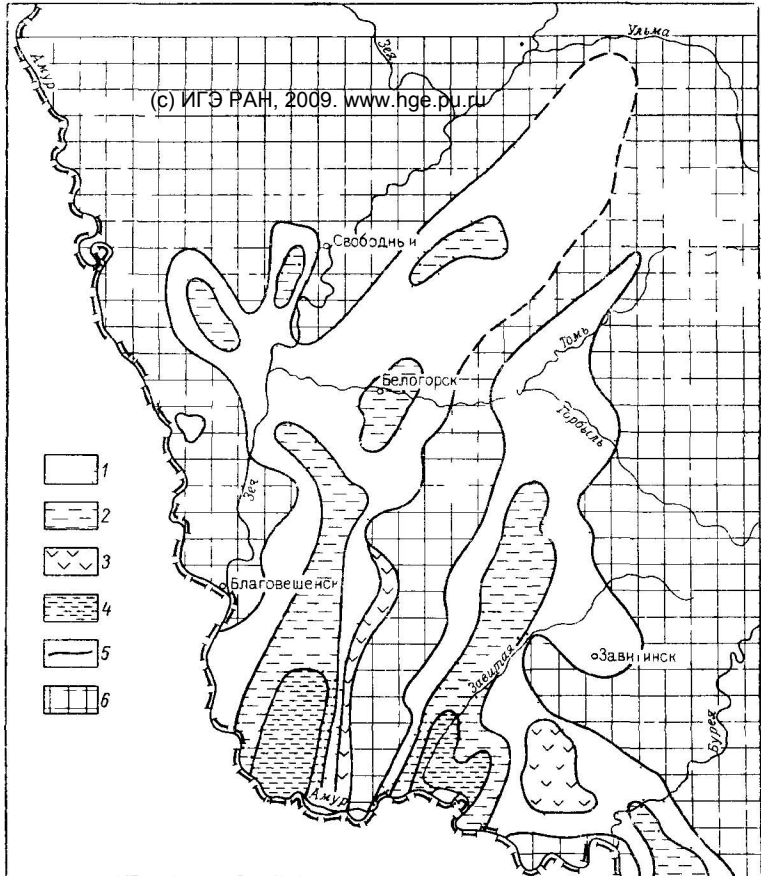
Рис 19. Схема распространения и характер водовмещающих пород водоносного комплекса нижнемеловых отложений (поирковская свита)
