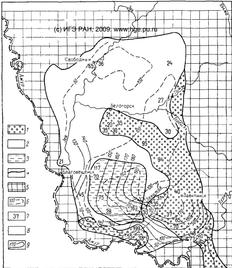
Рис 16. Схема распространения и характер водовещающих пород водоносного комплекса верхнемеловых отложений среднебайкальской подспиты. Подземные воды 1 — в мощных (до 20—40 м) пачках песков и гравия (иногда галечников) 2 — в песках с прослоями гравия, 3 — в маломощных пачках песков (иногда глинистых), залегающих среди глины и алевролитов 4 — граница распространения литологических комплексов пород 5 — районы отсутствия отложений подспиты 6 — изолинии мощности водоносного комплекса (м), 7 — мощность водоносных пород (м), 8 — участки распространения самоизливающихся подземных вод, 9 — гидронизопезы, абс м
