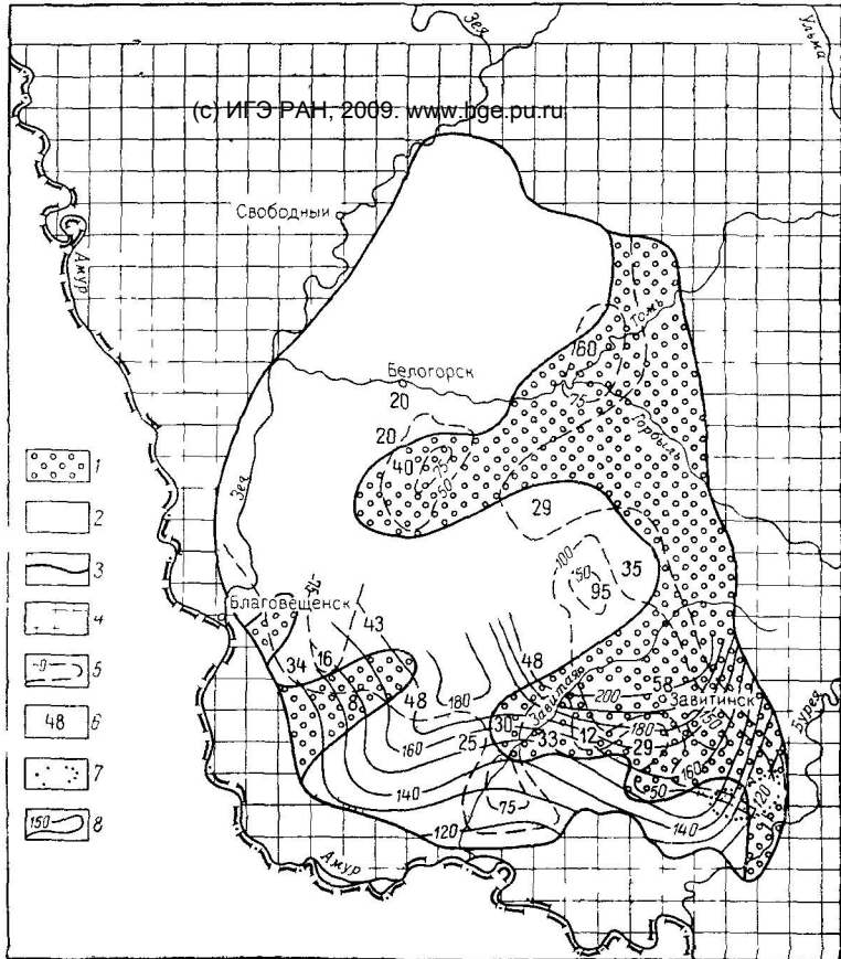
Рис. 15. Схема распространения и характер водовмещающих пород водоносного комплекса верхнемеловых отложений верхнецагайской подсвиты Подземные воды: 1 — в песчано-гравийно-галечниковых отложениях с маломощными прослоями глин, 2 — в песчаных (реже песчано-гравийных) отложениях с прослоями и пластинами глин и алевролитов; 3 — границы литологических комплексов пород; 4 — районы отсутствия отложений подсвиты; 5 — изопахиты водоносного комплекса (м); 6 — мощность водоносных пород (м); 7 — участки распространения самоизлывающихся подземных вод; 8 — гидрокзопезы, абс. м.
