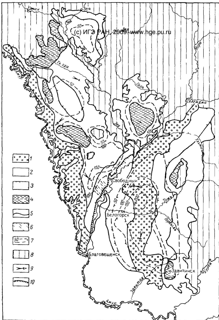
Рис 13 Схема распространения и характер водовмещающих пород водоносного горизонта миоценовых отложений (сазанковская свита)
