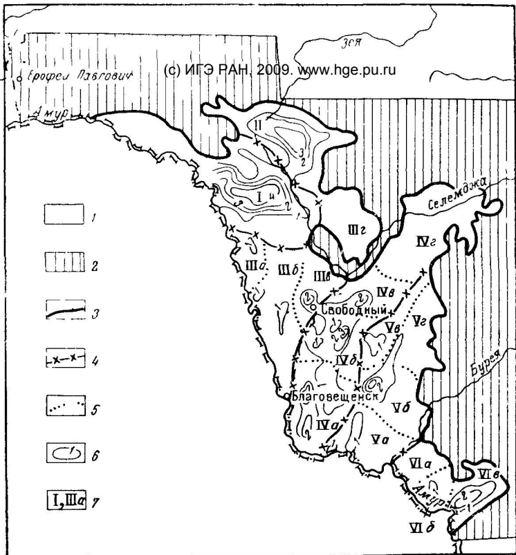
Рис. 11. Схема гидрогеологического районирования Амуро-Зейского артезианского бассейна
