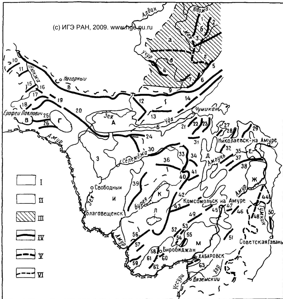
Рис. 1. Схема орографии Хабаровского края и Амурской области (по Ю. Ф. Чемякову, М. Н. Петрусевич и Н. С. Шапк)
