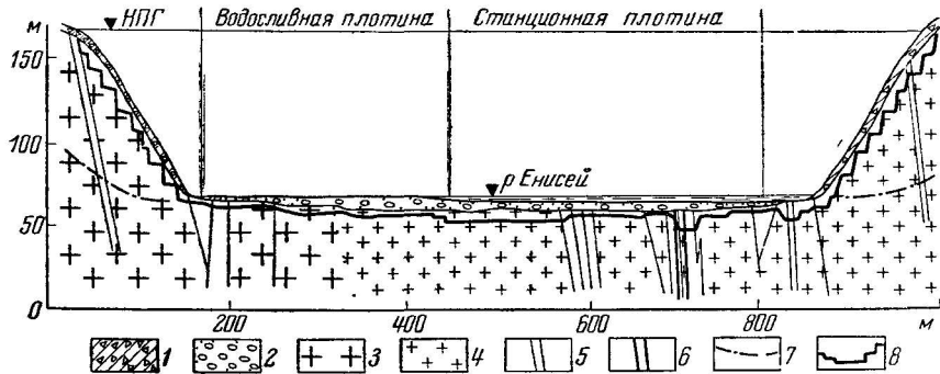
Рис. 70. Инженерно-геологический разрез по оси плотины Красноярской ГЭС 1 — делювиальные суглинки и щебень; 2 — аллювиальные галечники; 3 — граниты среднезернистые; 4 — граниты мелкозернистые; 5 — дайки порфиров, вогезитов, сиенитов, 6 — главная тектоническая зона; 7 — уровень подземных вод; 8 — врезка сооружения
