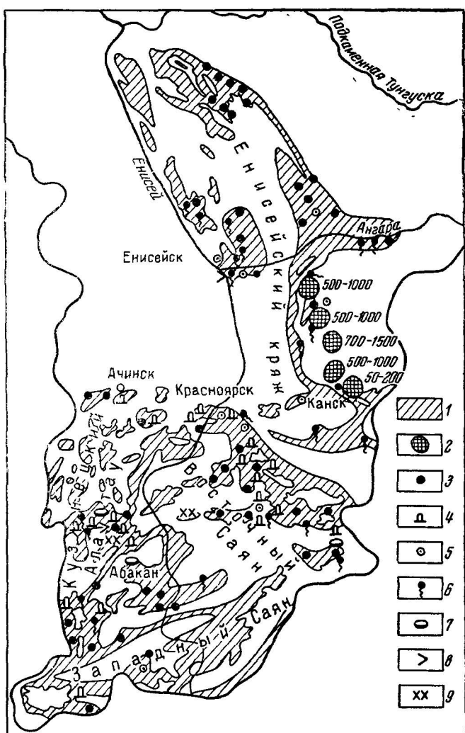
Рис. 68. Схема распространения закарстованных пород и карстовых явлений юга Красноярского края (по материалам Ж. Л. Цыкиной)
