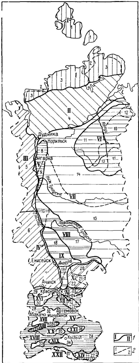
Рис. 65. Схема инженерно-геологического районирования. Составил А. А. Горюнов
