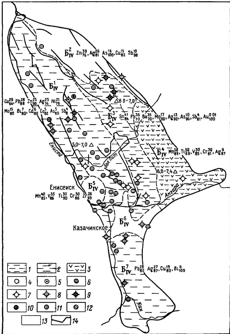
Рис 58 Схема гидрогеохимического прогноза на рудные и нерудные ископаемые Енисейской складчатой области Составил Н Г Шубенин
