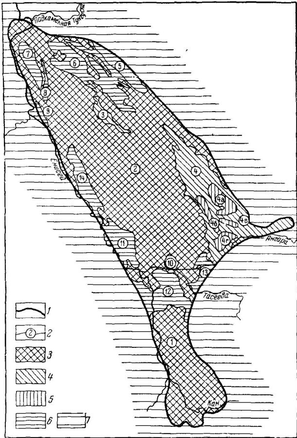
Рис. 38. Схема гидрогеологического районирования Енисейской складчатой области. Составили Л. Г. Заварзин и Н. Г. Шубенин
