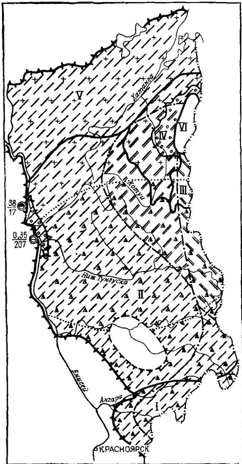
Рис. 37. Схематическая карта водоносности отложений верхнего протерозоя Восточно-Сибирской артезианской области. Составил Е. А. Басков Условные обозначения те же, что на рис. 24
