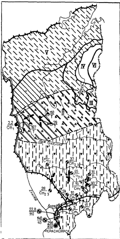
Рис. 36. Схематическая карта водоносности отложений нижнего отдела кембрийской системы Восточно-Сибирской артезианской области. Составил Е. А. Басков
