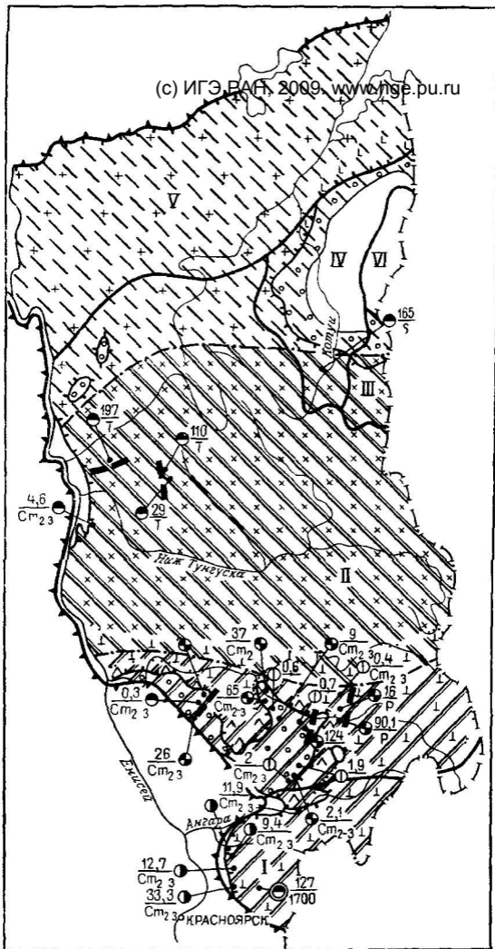
Рис. 35. Схематическая карта водоносности отложений верхнего и среднего отделов кембрийской системы Восточно-Сибирской артезианской области. Составил Е. А. Басков
