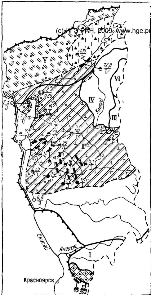
Рис. 31. Схематическая карта водоносности отложений девонской системы Восточно-Сибирской арзжанской области. Составил Е. А. Басков Условные обозначения те же, что на рис. 24
