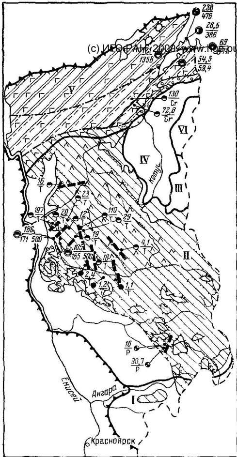
Рис. 27 Схематическая карта водоносности отложений пермской системы Восточно-Сибирской области. Составил Е. А. Басков
