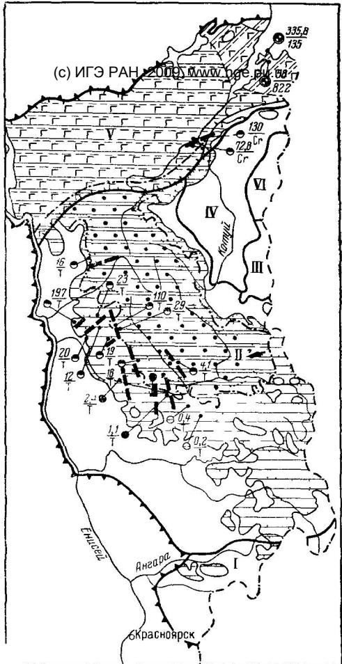
Рис. 26. Схематическая карта водоносности образований триасовой системы Восточно-Сибирской артезианской области. Составил Е. А. Басков Условные обозначения те же, что на рис. 24
