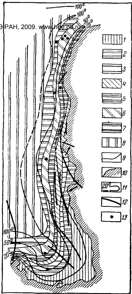
Рис. 23. Схематическая гидрохимическая карта подземных вод верхней части фундамента Западно-Сибирской артезианской области. Составила Л. Г. Учителева
