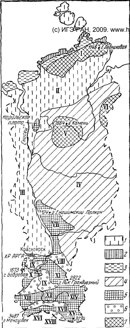
Рис 2. Схема рельефа (по Д. И. Мусатову)
