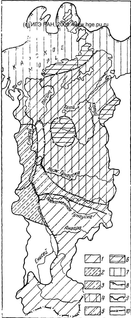
Рис. 18. Схема районирования территории региона по типам разрезов криогенной толщи. Составил С. М. Фотиев
