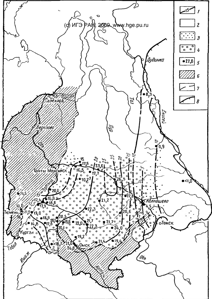
Рис. 33. Изменение минерализации и состава подземных вод нижней части готерив-барремских отложений (составили Б. П. Ставицкий, А. А. Розин)
