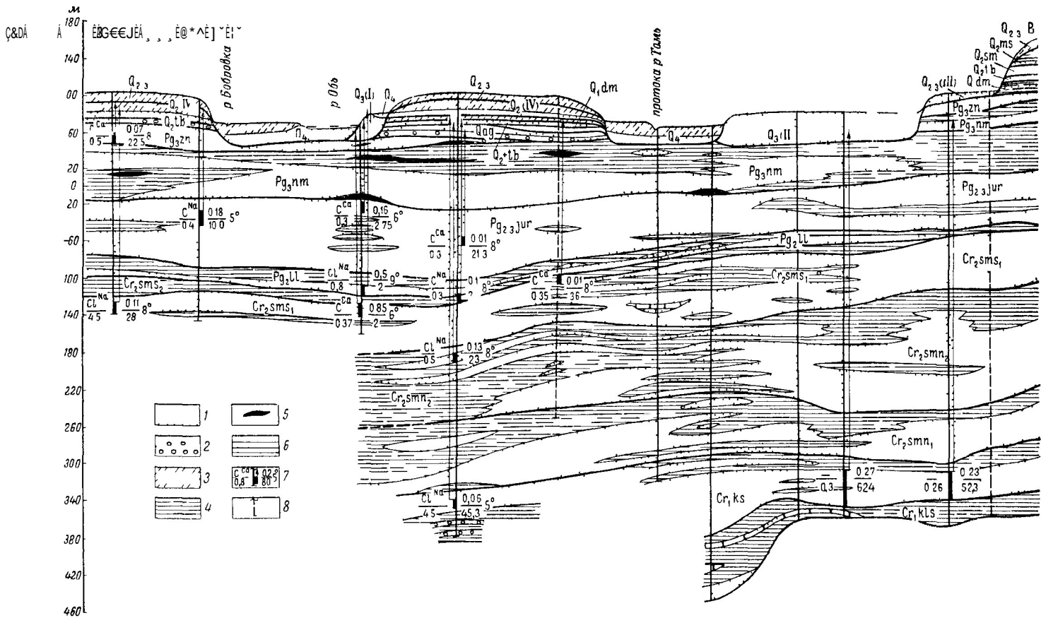
Рис. 18 Схематический гидрогеологический разрез Обь — Томского междуречья (составили Г. А. Чернышев и О. А. Гусельникова)
